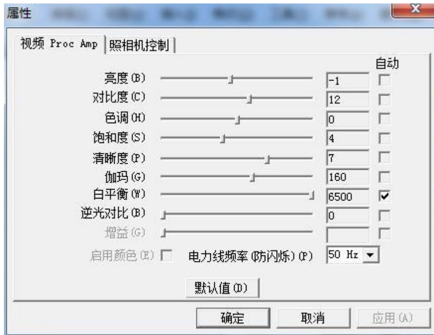
属性参数 (图 5)
