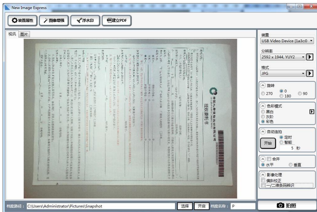
软件界面（图 1）
